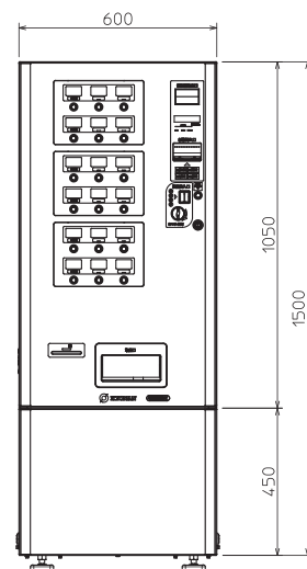
正面図
