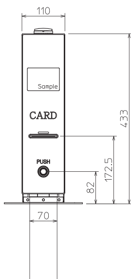
正面図
